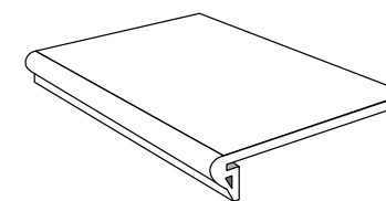
GRADINO CON TORO LARGHEZZA MAX 33 cm
